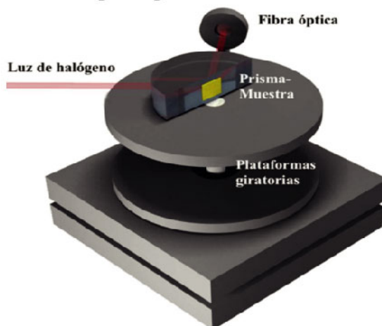
Figura 1. Diagrama del Sistema Experimental
